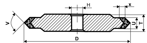
14EE1 D*T*U*X*V*H
