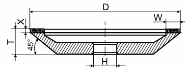
12A2-45° D*W*X*T*H
