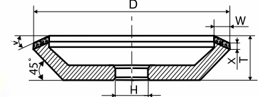
12V5-45° D*T*W*X*V*H
