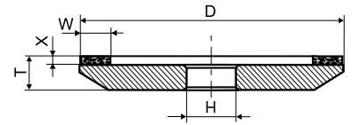
4A2 D*T*X*W*H
