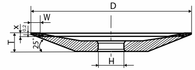
12R4 D*W*X*T*H
