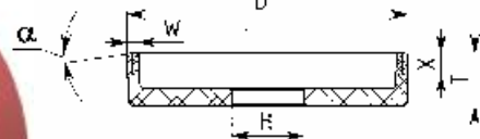
6A2 D*W*X*T*H*α°
