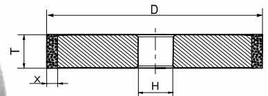
1A1 D*T*X*H
