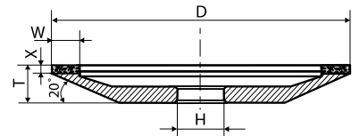
12A2-20° D*T*X*W*H
