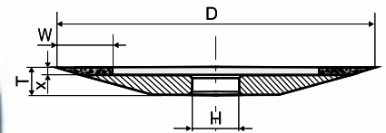
4B2 D*T*X*W*H
